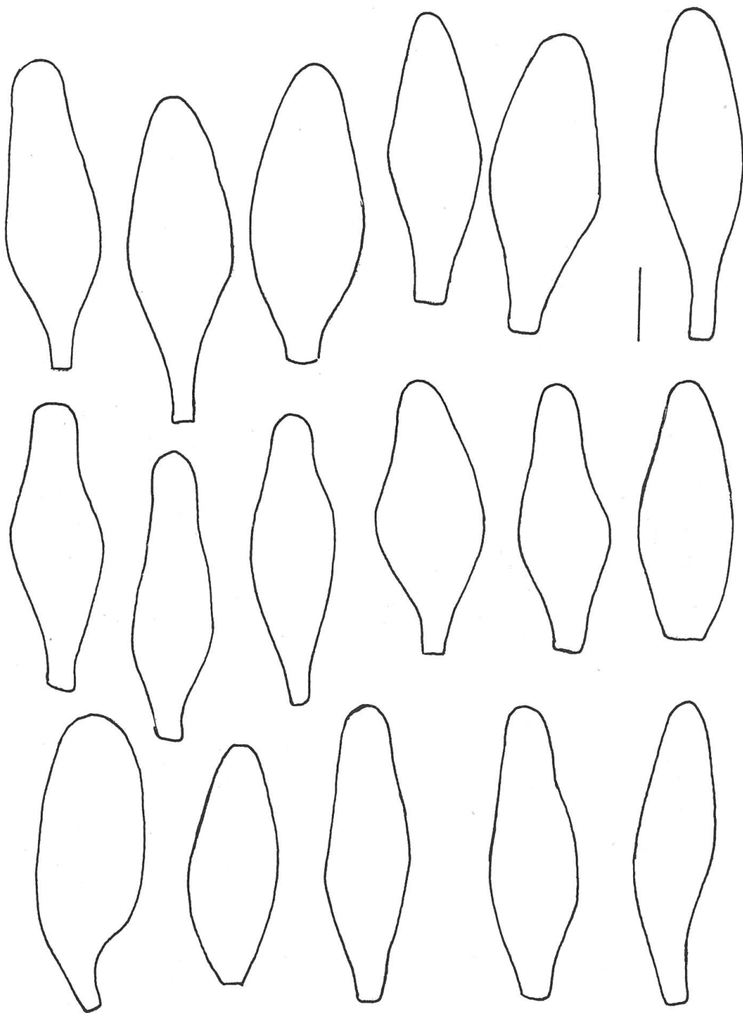
Fig. 2 : Pleurocystides
