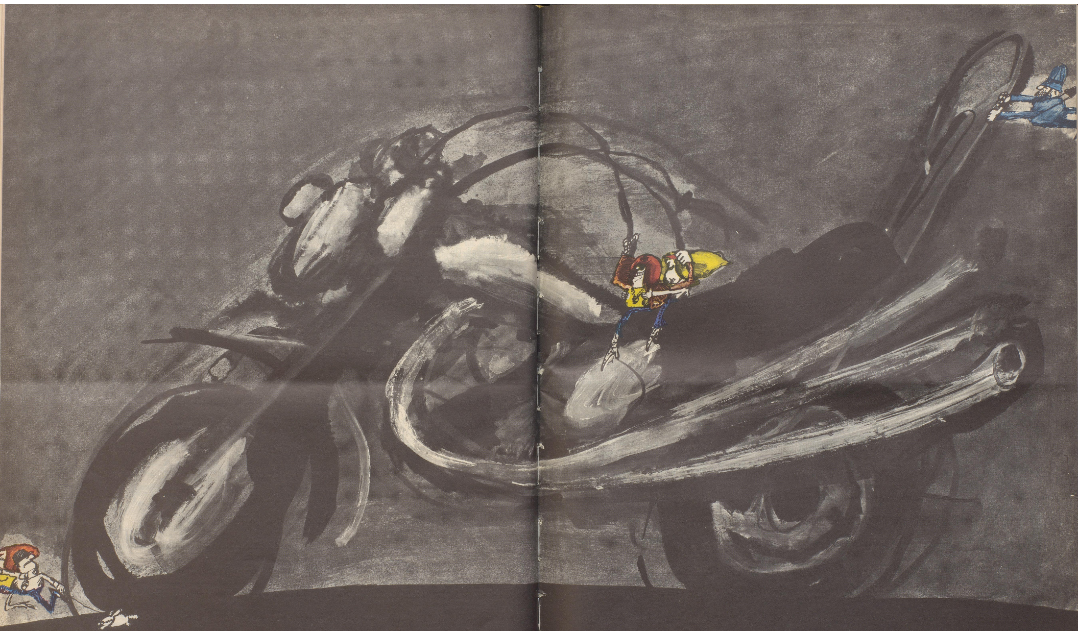
Das Kraftsymbol
