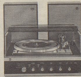
Dual HS 52. Hi-Fi-Automatikspieler Dual 1218, Hi-Fi-Verstärker 2 x 15 W, 2 Hi-Fi-Lautsprecher, Abdeck- haube. Tuner-, Tonband- und Kop- fhöreranschluss. Komplett in Nussbaum Fr. 1495.— In Weiss Fr. 1535.—
