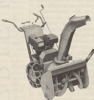
AEBI SF 1 8 PS, 65 cm Räumbreite
