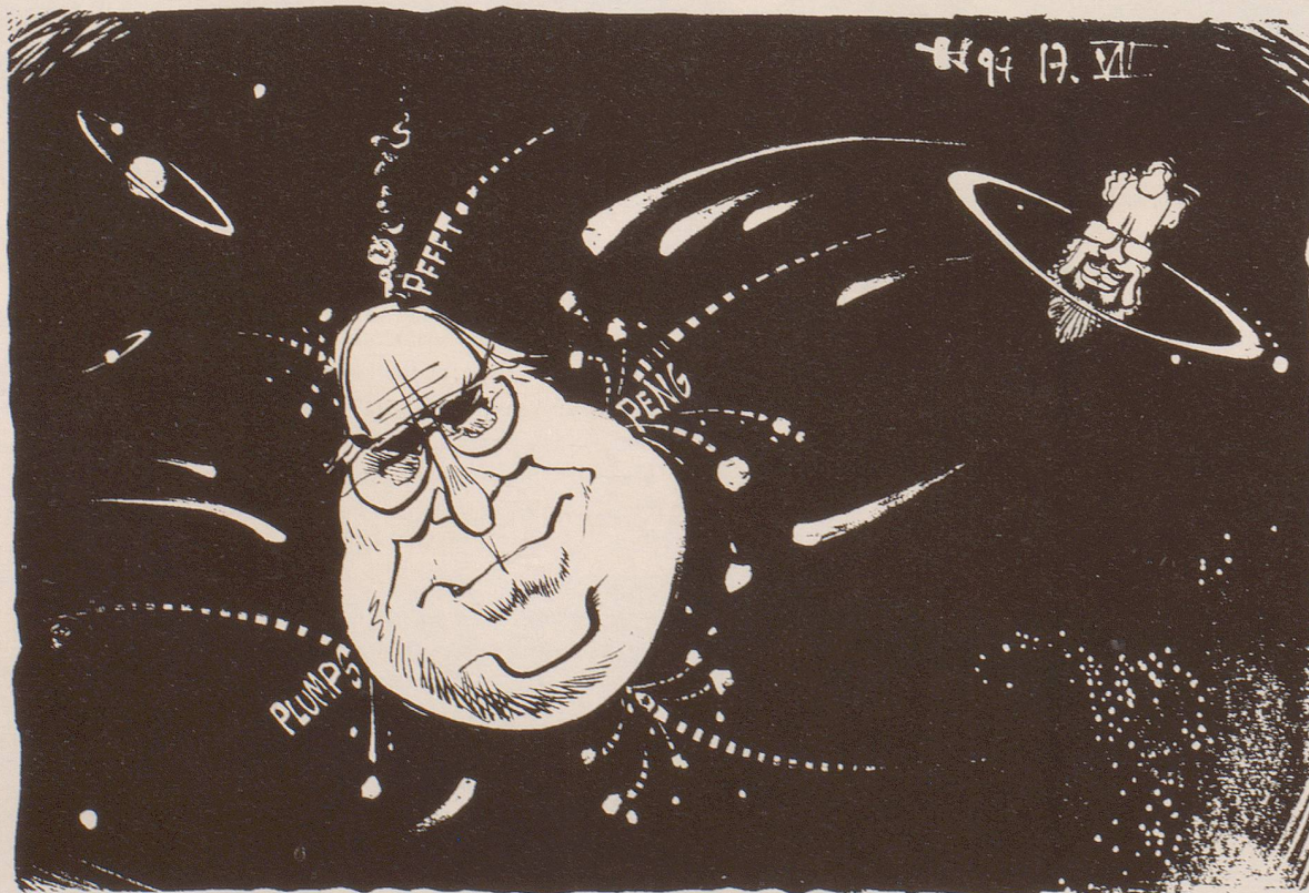
Jupiter, von Kometen attackiert
