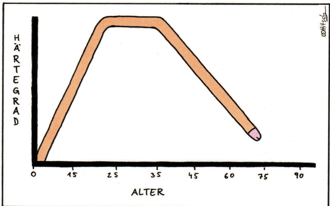
POTENZ - STATISTIK
