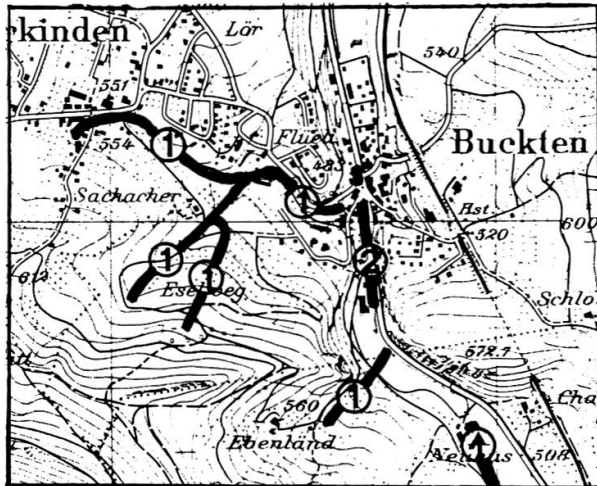
Abb. 10: Eindolungen im Raum Känerkinden/Buckten. Reproduziert mit Bewilligung des Eidg. Bundesamtes für Landestopographie vom 28. 3. 1988. 1: 1883–1955 eingedolte Gewässer. 2: 1955–1976 eingedolte Gewässer. Das Beispiel zeigt, dass das Gewässernetz ganzer Hänge flächenhaft eingedolt wurde.
