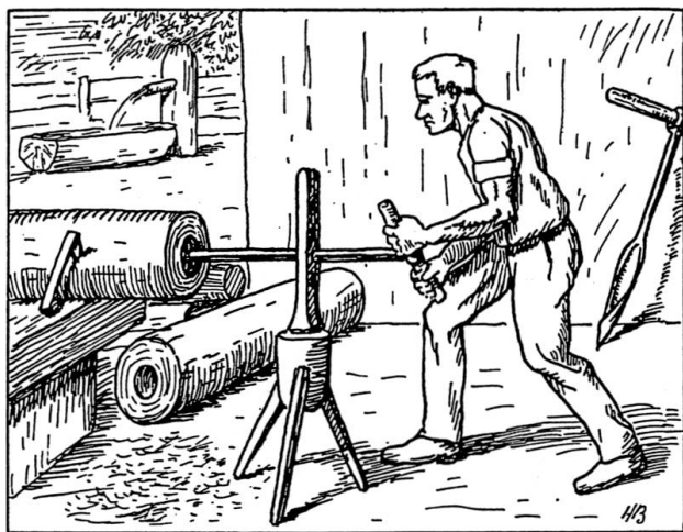
Abb. 2: Der Teuchelbohrer: Geeignete Föhren- und Lärchenstämme wurden auf oben gezeigte Weise zu «Teucheln» gebohrt. Beim Verlegen wurde in die Röhrenenden ein schmiedeeiserner Ring je zur Hälfte eingeschlagen und so die Leitung stabil verbunden und gedichtet. In gewissen Abständen hieb man kleine Schlitz in die Teuchel, die, durch Holzkeile abgedeckt, eine allfällige Kontrolle des Wasserlaufes ermöglichten. (Quelle: «Wasserversorgung Titterten», 1987, Gemeindearchiv)
