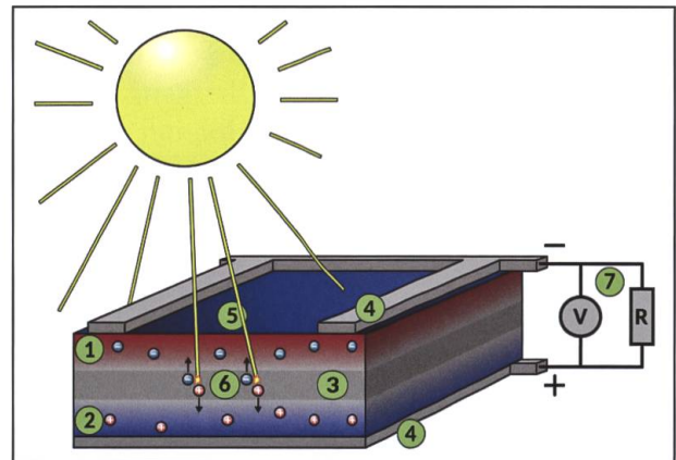
Abb. 7: Silizium-Photozellen zur Erzeugung von Solarstrom.
