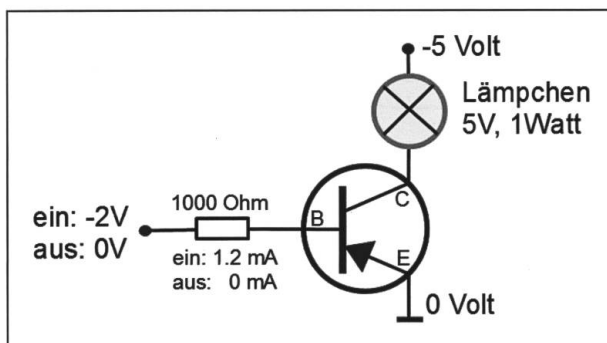
Abb. 15: Transistor als Schalter ersetzt Relais. Das 1-Watt-Lämpchen wird mit einem Strom von etwa 1,2 mA bei 2 Volt eingeschaltet. Die für das Einschalten aufzuwendende Leistung beträgt nur 2,4 mW, rund 400-mal weniger als das Lämpchen (Bild: Fritz Gassmann).
