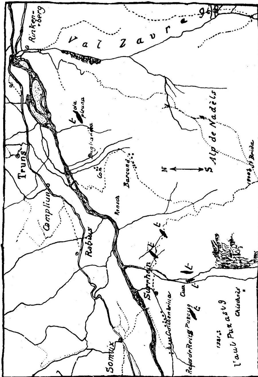
Fig. 2. Kärtchen der Umgebung von Surrhein-Somvix und Rinken-berg-Truns. (t = Lavezstein und Talkschiefer.)
