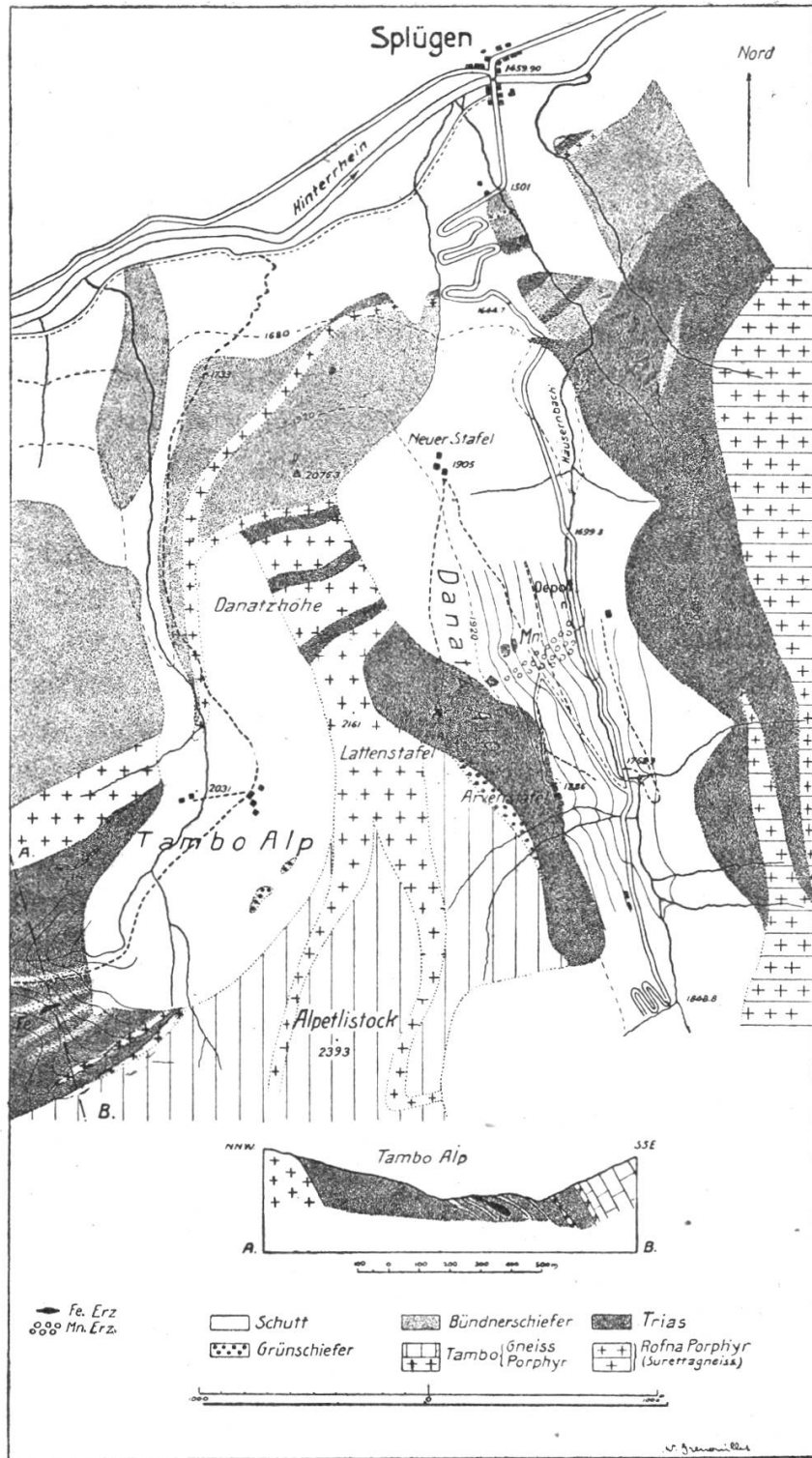
Fig. 5. Manganzvorkommen auf der Danatzalp.
