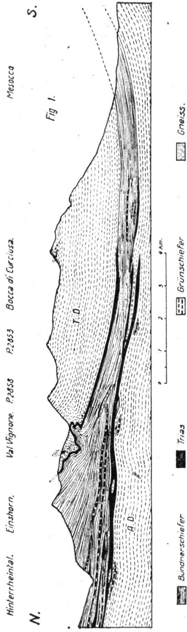
Fig. 1. Profil durch die Tamboeck.
