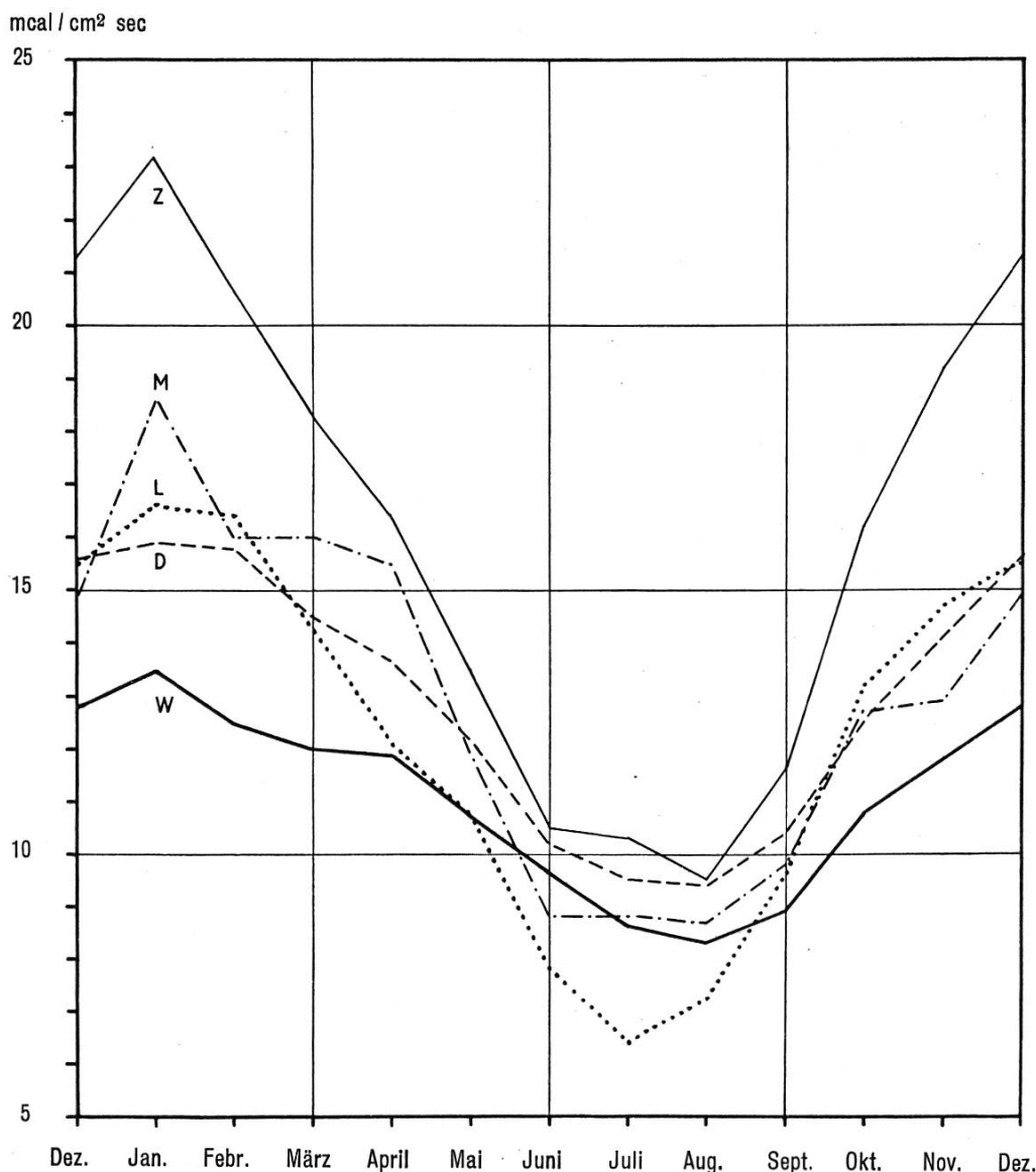
Abb. 6. Jahrgang der Abkühlungsgröße in mcal/cm 2 sec.
