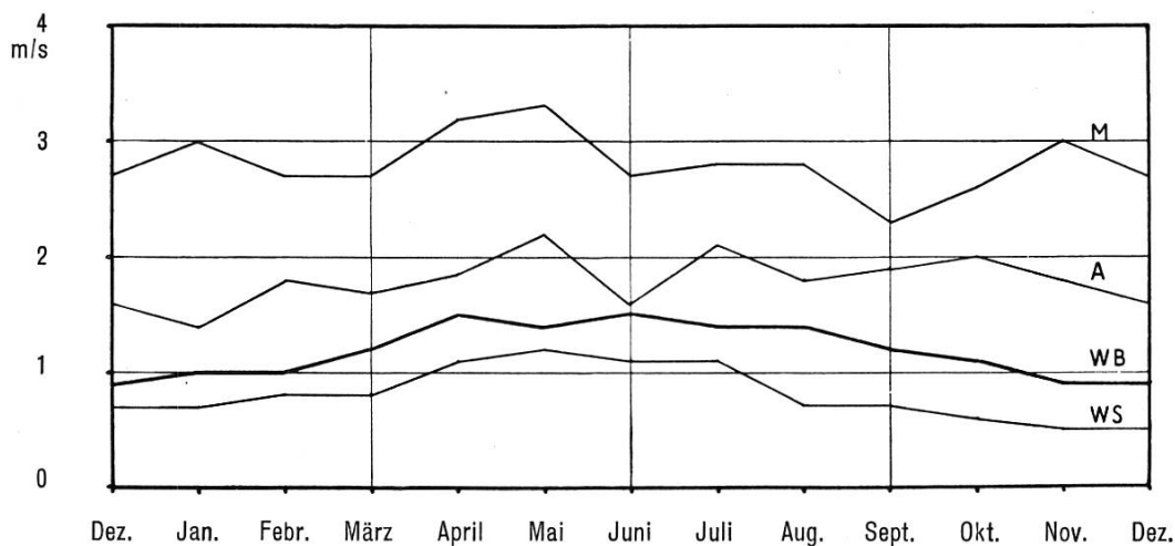
Abb. 5. Jahresgang der Windgeschwindigkeit in m/s. WB: Wiesen-«Bergruhe» Jahresmittel 1.2 m/s WS: Wiesen-«Sonnenhalde» Jahresmittel 0.8 m/s A: Arosa Jahresmittel 1.8 m/s M: Montana Jahresmittel 2.8 m/s
