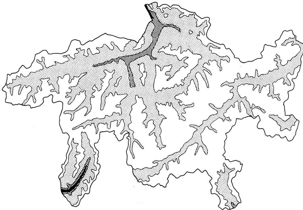
Abbildung 1: Die Höhengliederung des Kantons Graubünden, umgearbeitet nach IMHOF, Atlas der Schweiz 1965
