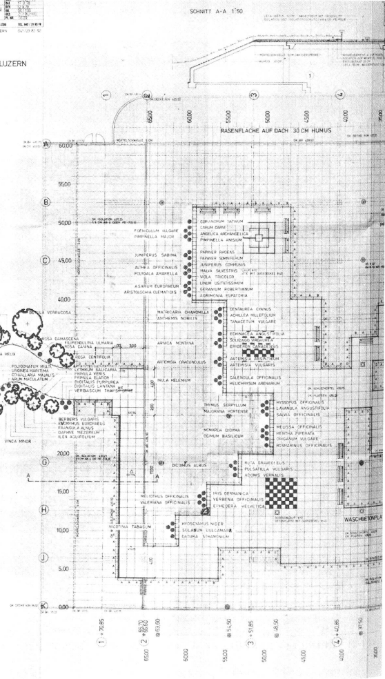
SNITT A-A 1:50
