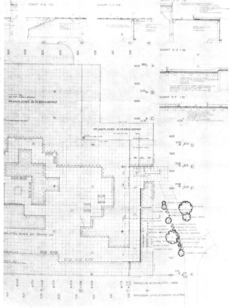
SNITT B-B 1:50
