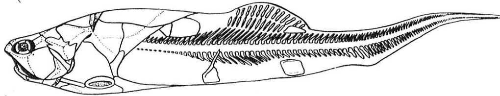
Coccosteus
