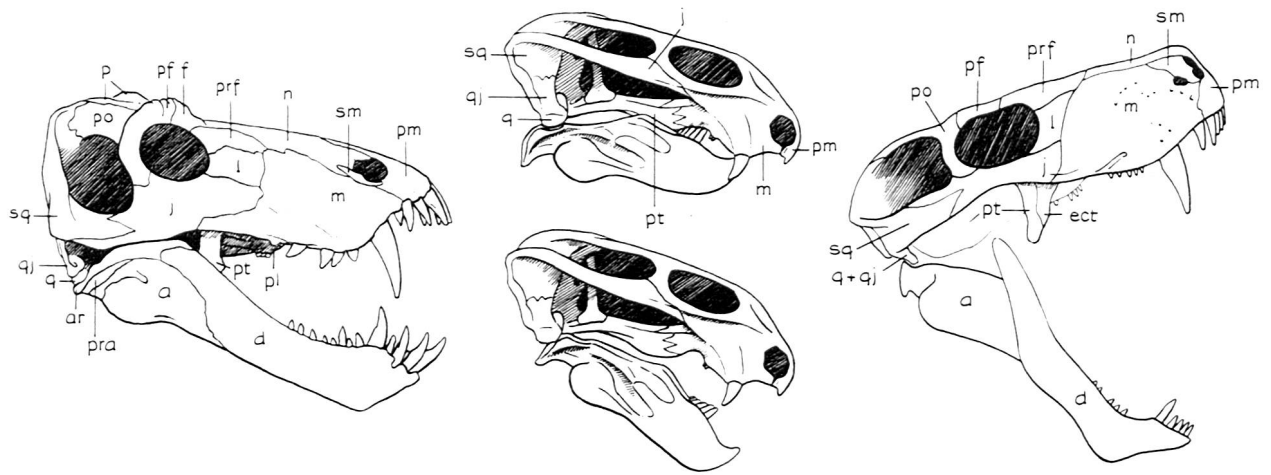
Titanophoneus
