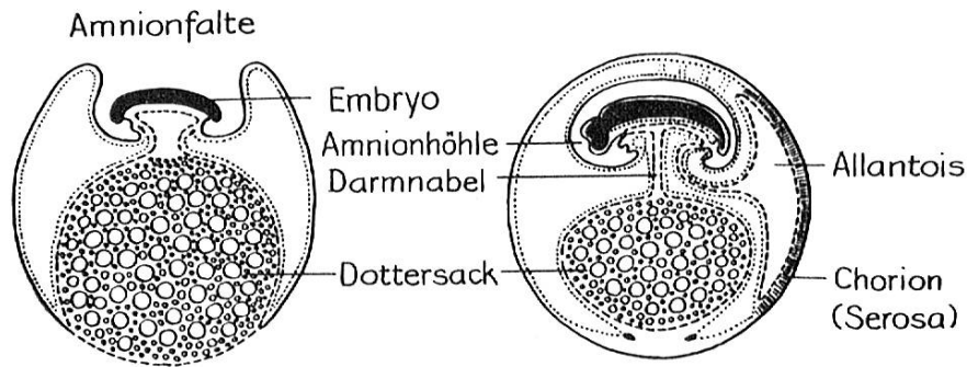
Abb. 50: Das Amniotenei.
