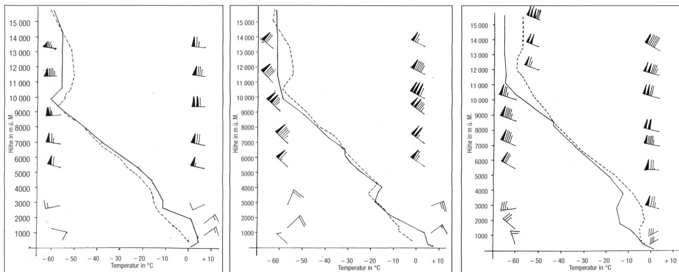
Abb. 7 Radiosondenaufstiege von Payerne (gestrichelt) und Mailand (ausgezogen) und den Höhenwinden, Windstärke in Knoten, über Payerne (rechts) und Mailand (links).
