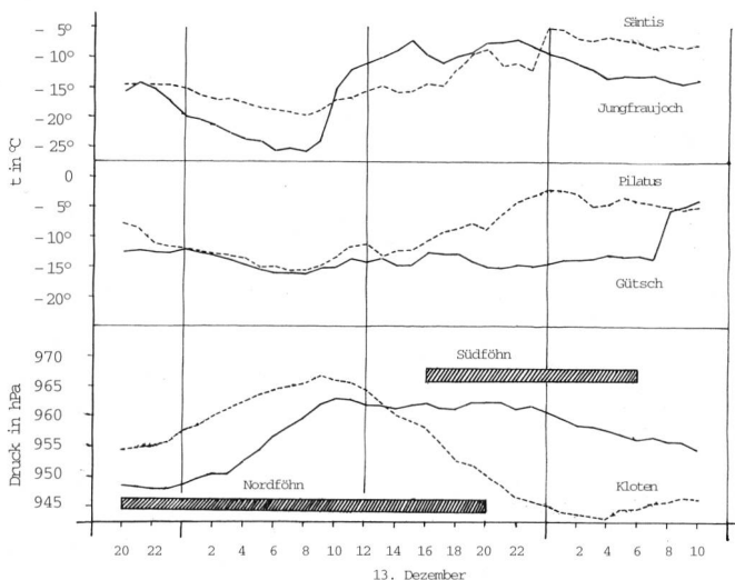
Abb. 6. Der Nord-Süd Gradienten des Luftdruckes zwischen Kloten und Locarno Monti (bezogen auf 400 m ü.M.) und der Temperaturverlauf an den Bergstationen Jungfrauoch (3572 m ü.M.), Säntis (2490 m ü.M.), Güttsch (2287 m ü.M.) und Pilatus 2106 m ü.M.)
