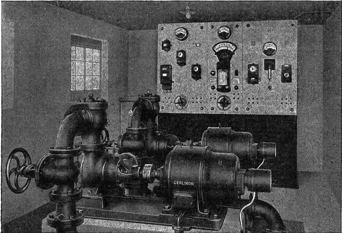
Automatische Pumpen-Anlage einer Wasserversorgung.
