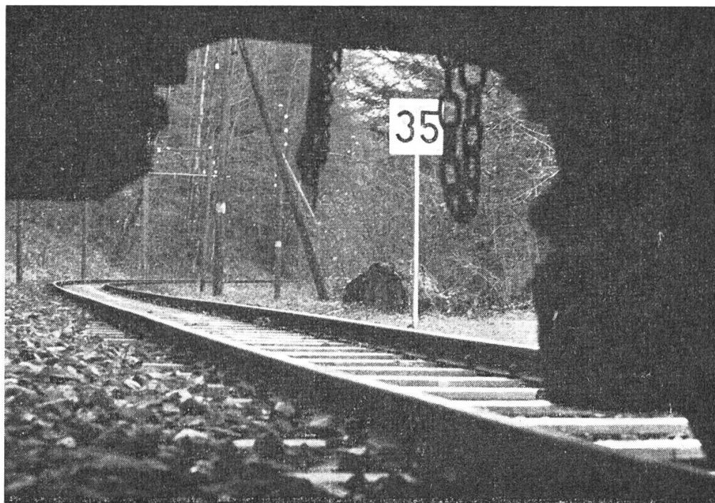
Die Kurven der Strecke Stansstad-Engelberg werden im Zuge der technischen Erneuerung gestreckt, um die Maximalgeschwindigkeit von 75 km/h wenn immer möglich ausnützen zu können.
