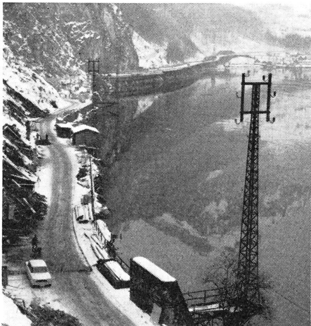
Im Januar 1965 die alte Lopperstrasse vom Portal des Tunnels Nord aus. Am Berghang sieht man die ersten Fundamente für das Lehnenviadukt vom Buchenloch.
