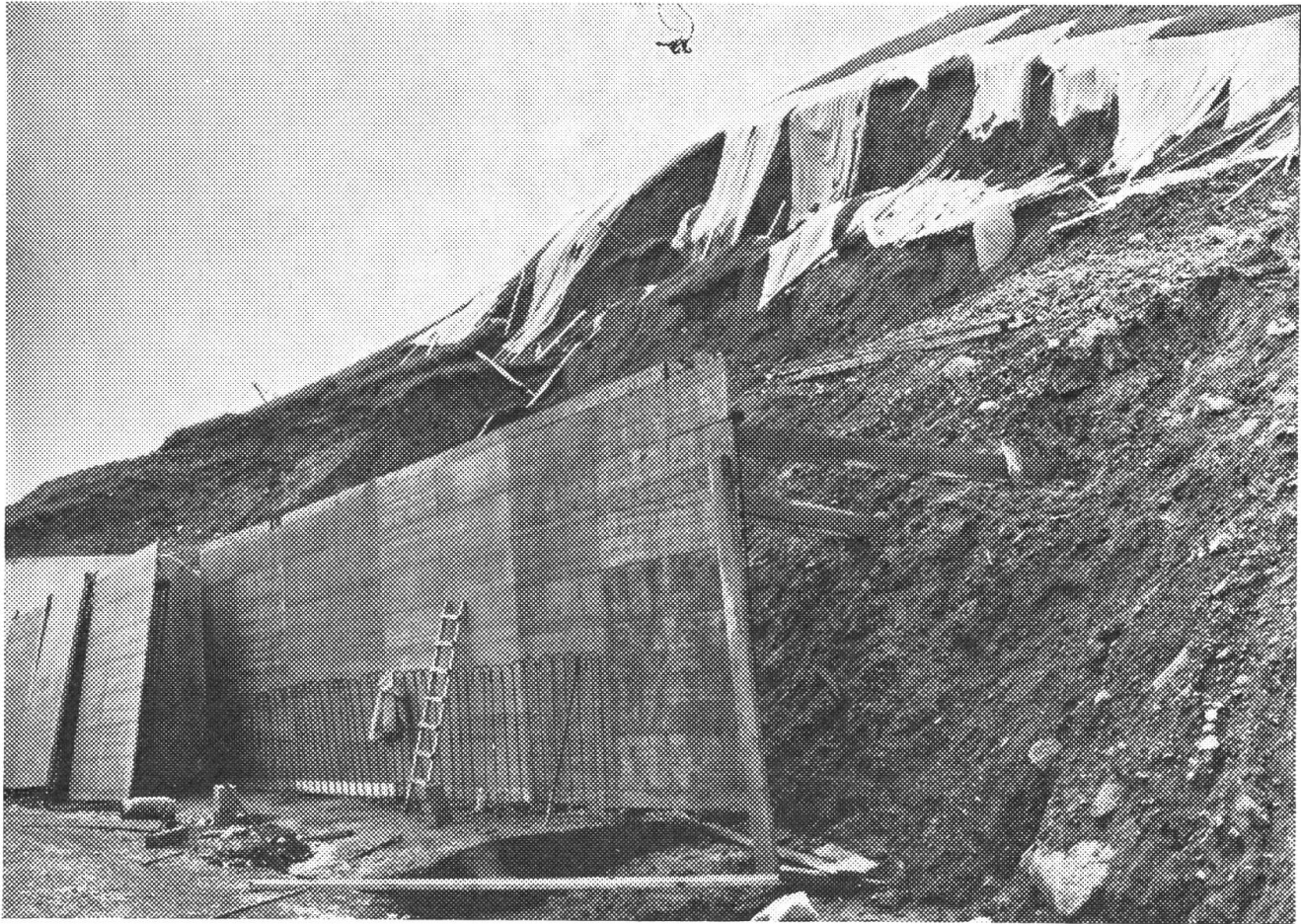
Solche Schwierigkeiten in durchnässter Hanglage gab es im Bauabschnitt Buochs. Um den noch größeren Schwierigkeiten im Rutschgebiet bei Bauen auszuweichen wurde die N 2 zwischen Beckenried und Seedorf neu konzipiert. Nach der neuen Linienführung wird zwischen Rütene-Beckenried und Bolzbach-Seedorf ein Tunnel von 9,2 km erstellt. Foto A. Odermatt
