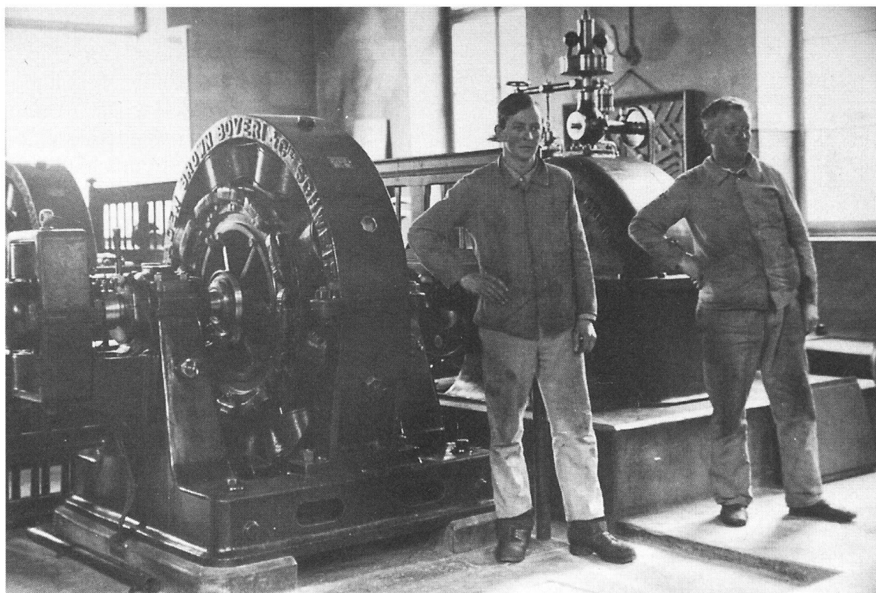
Zentrale Mühlebach, erbaut 1936, mit einem Wechselstromgenerator BBC 125 KVA 3150 Volt 48 Hz – Freistrahlf Pelton Turbinen, davor Werner Wymann, der Elektromonteur und Adolf Feller, der Maschinist.
