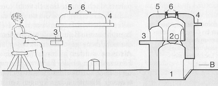
Schematische Darstellung eines Glasofens aus Avenches: B Feuerloch 1 Brennkammer, 2 Schmelzkammer, 3 Arbeitsfläche vor dem Zugang zum geschmolzenen Glas mittels der Glaspfeife, 4 Abstelltafel zum Auskühlen der fertigen Gefässe, 5 Kuppel, 6 verschliessbare Öffnungen zur Temperaturregulierung Nach Amrein 2001
