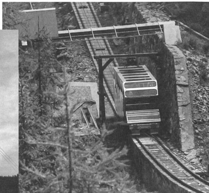
Standseilbahn Le Châtelard – Les Montuieres, Le Châtelard (VS), von Von Roll (1919). Wagen in Wannensegment mit Seil-Niederhalte-Joch und vorgelagertem Ballastwagen.
