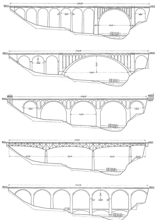
Abb. 2: Entwürfe für den Zähringerviadukt in Fribourg, 1923. Zuunster der zur Ausführung bestimmte Entwurf © SBZ, Band 81/16: 191
