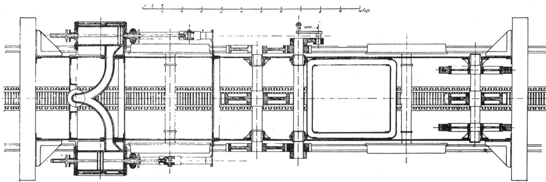
Bild 7 Projekt einer Lokomotive mit Zahnrad für die Überschienung der Alpen nach Riggenbach 1868
