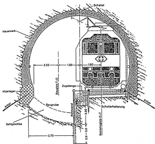
Die Rekonstruktion des Hauenstein-Basistunnels 1980–1987 mit Aufrechterhaltung eines eingleisigen Betriebes
