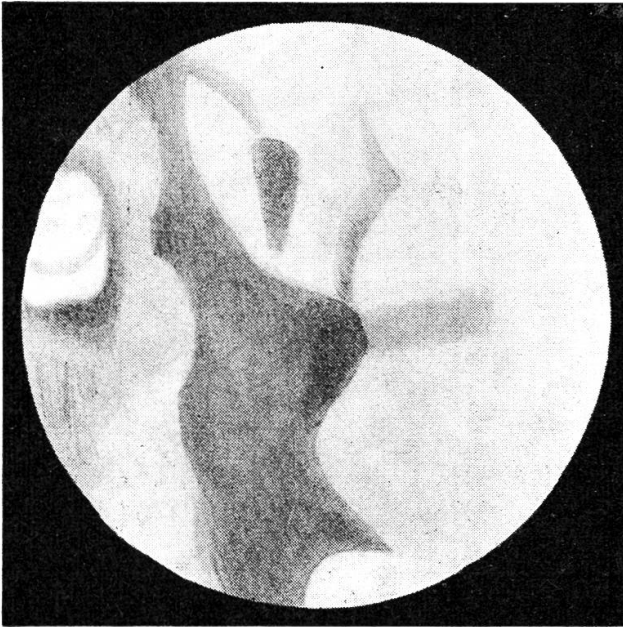
⑥ Août 28, 23 h. 55 \omega = 50^{\circ}, 4 , \varphi = -19^{\circ}, 1 , D = 24'' , 3 . \eta = 340^{\circ} . 220 \times . Im. = 4-5.
