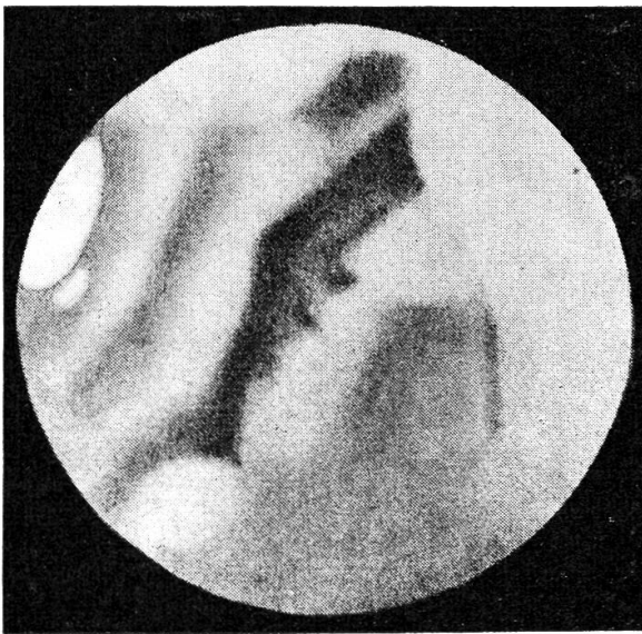
⑤ Août 16, 1 h. 40 \omega = 192^{\circ}, 6 , \varphi = -19^{\circ}, 4 , D = 22'' , 8 . Ph = 0'' , 9 , \eta = 332^{\circ} . 220 \times . Im. = 5-6.
