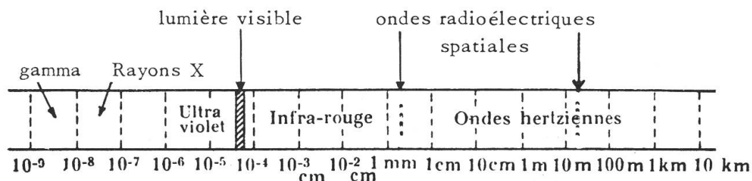
Figure 2 – Spectre électromagnétique.
