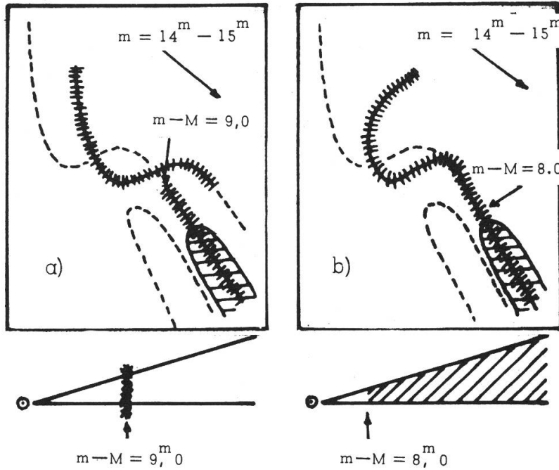
Abbildungen 13a und 13b – Schematische fraktionierte Zweifarbenindexdiagramme mit Verfärbungseinflüssen bei a) Absorptionsschirm mit Entfernungsmodul 9.^m_0 , b) gleichmässiger Absorption, beginnend mit dem Entfernungsmodul 8.^m_0 . Besetzung durch Zwerge eng schraffiert, durch Riesen weit schraffiert (nach W. Becker und U. Steinlin).
