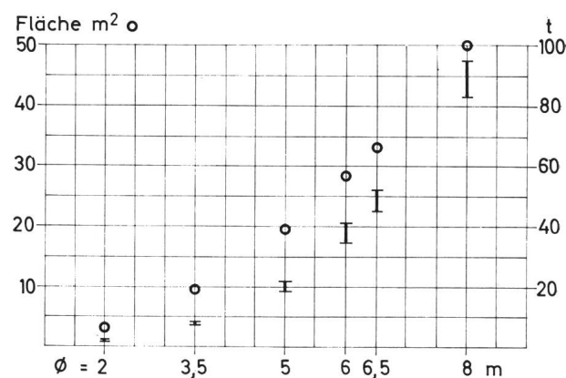
Teleskopspiegel Skelett-Bauweise
