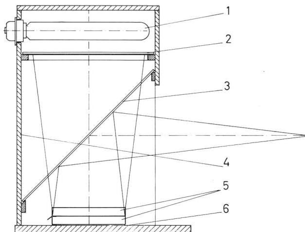
Abb. 3: Kontroll-Vorrichtung im Schnitt: 1. Natriumdampflampe, zweckmässig mit einem Aluminium-Reflektor überdeckt; 2. Opalglasscheibe; 3. Klarglasscheibe; 4. mattschwarze Rückwand; 5. Planspiegel, links Alu-Zwischenlage; 6. mattschwarze Unterlage. Die Betrachtung der Spiegel soll aus wesentlich grösserer Entfernung (ca. 10 \times Spiegeldurchmesser) erfolgen als auf der Skizze angedeutet.
