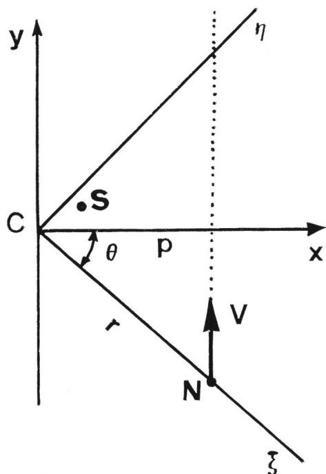
Fig. 3: Passage d'un nuage de centre N et de vitesse V à proximité d'un amas stellaire de centre C.
