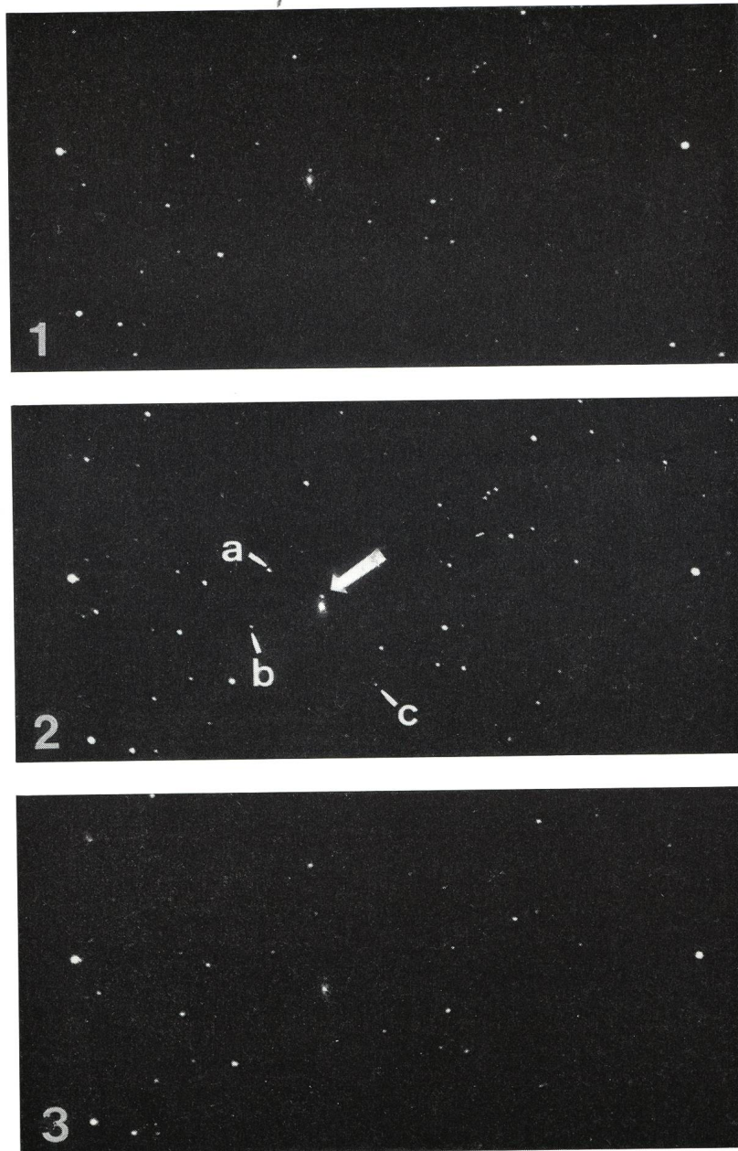
Fig. 1: 3 Aufnahmen von E. HEISER, Osnabrück mit Zeiss-Spiegellinsen-Objektiv (Mirotar) 1:4, f = 500 mm auf Kodak 103 a F-Film am 9. 5. 1974, 22 h 42– 22 h 52 MEZ, am 15. 5. 1974, 23 h 55–24 h 00 MEZ und am
