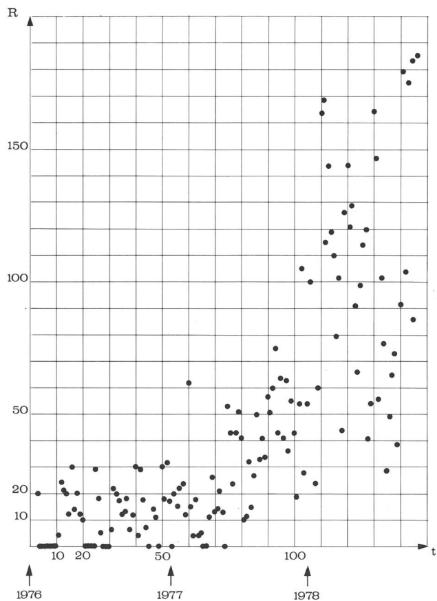
Graphische Darstellung (Wochenmittel), bei der die Sonnenfleckenrelativzahl R gegen die Zeit in Wochenabständen aufgetragen ist. Etwa Mitte 1977 ist der Zuwachs deutlich erkennbar, 1978 nimmt R besonders rasch zu.
