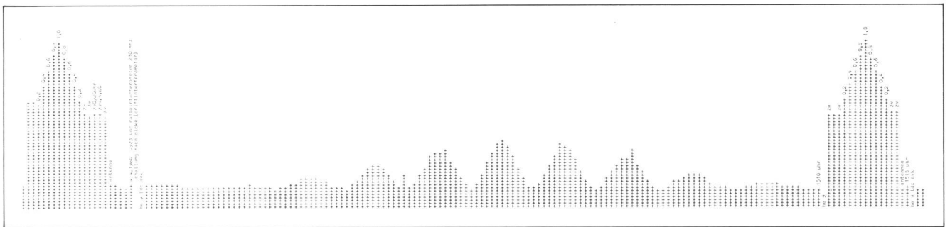
Abb. 9: Interferogramm der solaren Radiostrahlung, aufgezeichnet mit dem mikroprozessorgesteuerten Fernschreiber Lorenz 15. Am Anfang und am Ende ist je eine kalibrierte Rauschtrepppe aufgedruckt mit einem maximalen Zusatzrauschen von 300 Kelvin ( 1T_0 ).
