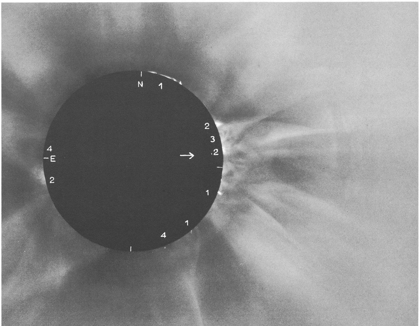
Fig. 2. Die innere Korona, aufgenommen im blauen Licht ( \lambda_{\text{eff}} = 440 \text{ nm} ) 30^{\text{s}} vor 3. Kontakt. Belichtungszeit 16.5^{\text{s}} 1 = Protuberanz, 2 = Kondensation, 3 = koronale Bögen, 4 = Kavität. Kondensationen sind heisse, dichte Gebiete über aktiven Regionen. In der dreieckigen Kondensation auf der Westseite liegt ein sehr heller Bogen, die hellste Struktur dieser Korona. Die hellen und dunklen Bögen repräsentieren geschlossene Magnetfelder. Die Kavitäten sind Zonen geringer Dichte am Fuss der langen Koronastrahlen, die über den Trennlinien von Magnetfeldregionen verschiedener Polarität liegen. In der mit Pfeil bezeichneten Region sind gegenüber Aufnahmen aus Ostafrika, die zwei Stunden früher gemacht wurden, in der inneren und äusseren Korona bedeutende Änderungen festzustellen. (Vergl. dazu Sky and Telescope , Mai 1980.)
