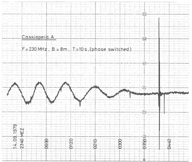
Abb. 8: Interferenzradiosignal verursacht durch den Supernova-überrest CASSIOPEIA A. Der Milchstrassenhintergrund ist elektronisch ausgeblendet, damit die Punktquelle CASS. A besser dargestellt werden kann. Rechts aussen starke elektr. Störung.
