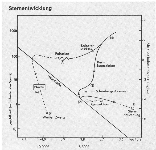
Abb. 1: Hertzsprung-Russell-Diagramm.
