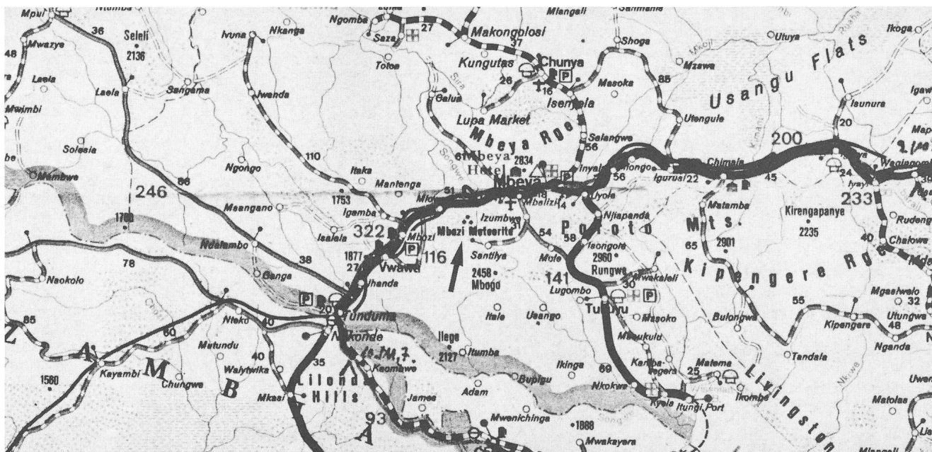
Abb. 3: Ausschnitt aus der Strassenkarte von Tanzania (1:2 000 000). Die mit drei Punkten angegebene Lage des Meteoriten stimmt nicht ganz. Er befindet sich etwas weiter südwestlich, ungefähr bei der km-Zahl «116» links vom Pfeil.
