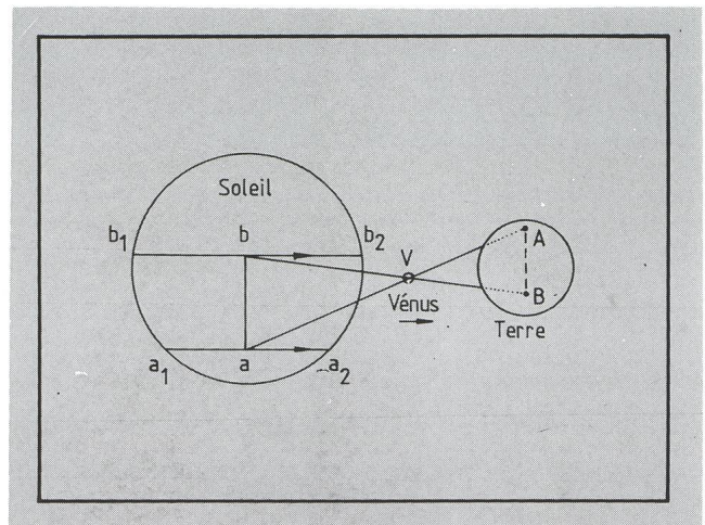
Mesure de la distance solaire par la méthode de Halley: Deux observateurs, A et B, placés sur la Terre à des latitudes différentes, voient passer Vénus devant le disque solaire selon deux cordes a_1 a_2 et b_1 b_2 , dont les longueurs sont proportionnelles aux temps de passage. On en déduit la distance ab relative au diamètre apparent (connu) du disque solaire. Le lien entre les triangles semblables Vab et VAB est donné par la 3 é loi de Kepler en utilisant les périodes (connues) de Vénus et de la Terre. La distance AB étant connue, on en déduit le diamètre du Soleil, d'où aussi sa distance.
