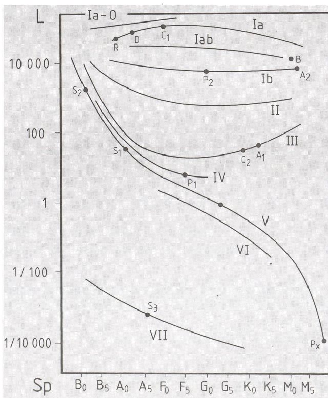
Figure 5: Les classes de luminosité. ○ désigne le Soleil (spectre G2 V) R: Rigel; D: Deneb; C1: Canopus; B: Bételgeuse; P2: l'étoile Polaire; A2: Antarès; C2: Capella; A1: Arcturus; S2: Spica; S1: Sirius A; P1: Procyon; Px: Proxima; S3: Sirius B. En ordonnée, on a remplacé la magnitude absolue par la luminosité intrinsèque, celle du Soleil étant prise comme unité.
