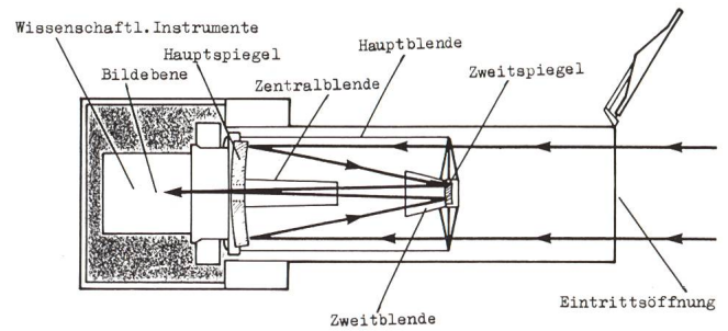
Abb. 1. Das Hubble-Teleskop
