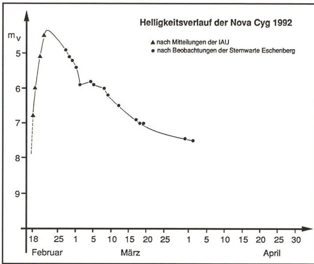
Bild 2 Hier die im steilen Anstieg aus einigen IAU-Werten und den zahlreichen Beobachtungen der Sternwarte Eschenberg abgeleitete Helligkeitskurve. In den ersten Märztagen zeigte sich eine in der abklingenden Phase von Novae sehr typische Flackerphase.
