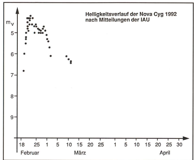
Bild 3 Die in dieser Graphik dargestellten visuellen Helligkeitswerte wurden den IAU-Zirkularen entnommen. Sie zeigen streckenweise eine verblüffend grosse Streuung, zum Teil aber auch die guten Übereinstimmungen mehrerer Beobachter.
