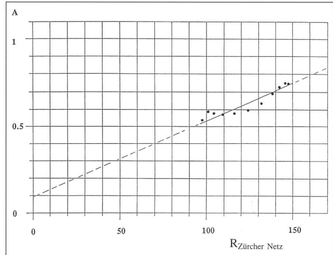
Bild 2: Übereinstimmung von A_{Ta} zu R_{Zürcher} Netz von August 1991 bis Juni 1992 R_z = -19,0 + 225,0 A_{Ta}
