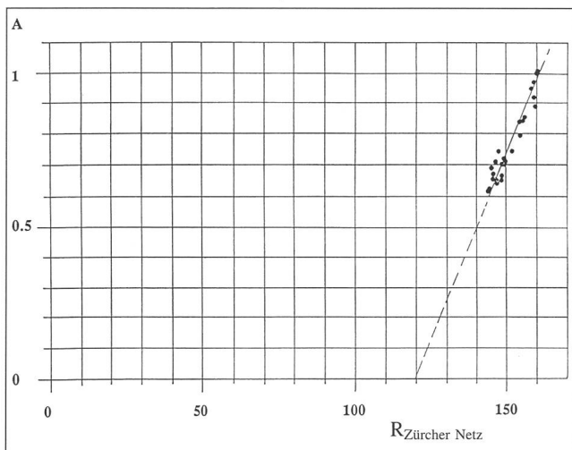
Bild 1: Übereinstimmung von A_{Ta} zu R_{Zürcher} Netz von Juni 1989 bis August 1990 Nach dem Maximum Korrelationsfaktor = 0.956 R_z = 119,6 + 41,2 A_{Ta}
