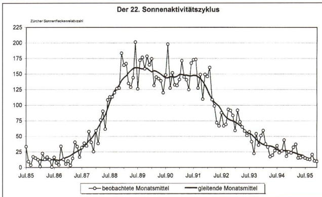
Abb. 1: Zürcher Sonnenfleckenzahlen 1985 - 1995
