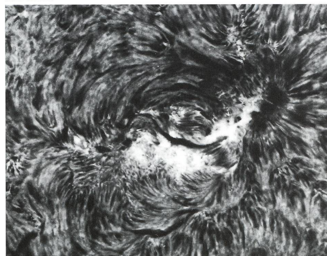
Abbildung 8: Sonnenfleck im H-alpha-Licht. 7. Oktober 1993. 12" Chromat. Äquivalentbrennweite 12,5 m, DayStar Filter 0,05 nm HWB, \frac{1}{60} s auf TP 2415. Die kleinen Flecken der Gruppe sind von Flares und Surges überdeckt.
