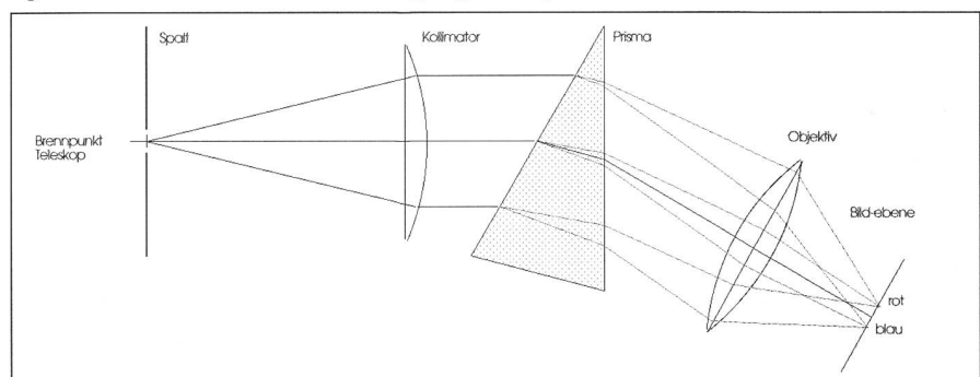
Fig. 1: Schematischer Aufbau zur Erzeugung eines Spektrums
