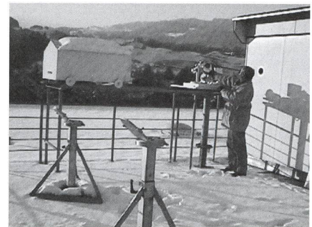
Fig. 2: W. WINIGER am Coelostat mit 10cm Spiegeln und abgefahrenem Gehäuse mit Blick nach Westen (Haus Gust). Das Sonnenbild von ca. 40cm Durchmesser wird durch ein liegendes Fernrohr von 160cm Brennweite und einem Spezialokular an der gegenüberliegenden Innenwand erzeugt. Gut sichtbar sind auch Details der in der Höhe verstellbaren Montierungen für 4 SC's. Man beachte auch die höchst reizvolle Landschaft.
