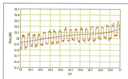
Fig. 3: Bestimmung des mittleren Mondradioflusses in Dezibel durch Einsatz einer Fitfunktion, um den Hintergrund vom Mondsignal zu trennen. Der langsam veränderliche Hintergrund auf Grund von veränderlicher Position und auf Grund schwankender Temperaturen im LNC und im Empfänger muss wegkompensiert werden. Die durchgezogene Kurve wird daher punktweise von der gestrichelten Fitkurve subtrahiert. Die statistische Untersuchung (Medianwert) des Differenzsignals führt zu einem einzelnen Flusswert, hier im Beispiel vom 16. Februar 2001 etwa 0.2dB. Die Fitkurve wird so bestimmt, dass die Streuung des Residuums ein Minimum wird. In vorliegendem Beispiel wurde ein Fitpolynom 4ten Grades verwendet.
