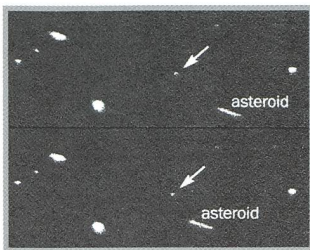
Les résonances gravitationnelles dans le système solaire - 4
