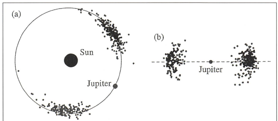
Fig. 2. Distribution des astéroïdes de Troyes sur l'orbite de Jupiter, le 18 décembre 1997 à 0^h UT. En (a) les astéroïdes sont projetés sur le plan de l'écliptique, en (b) ils sont vus le long de l'axe Jupiter-Soleil et la ligne en tirets représente l'orbite de la planète. (repris de [1])
